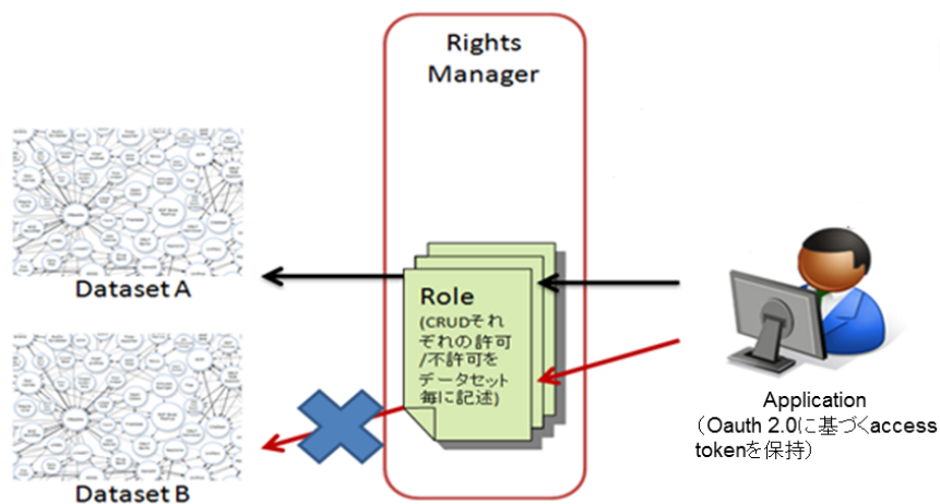
図 4.1: Security Management Command によるアクセス制御のイメージ
