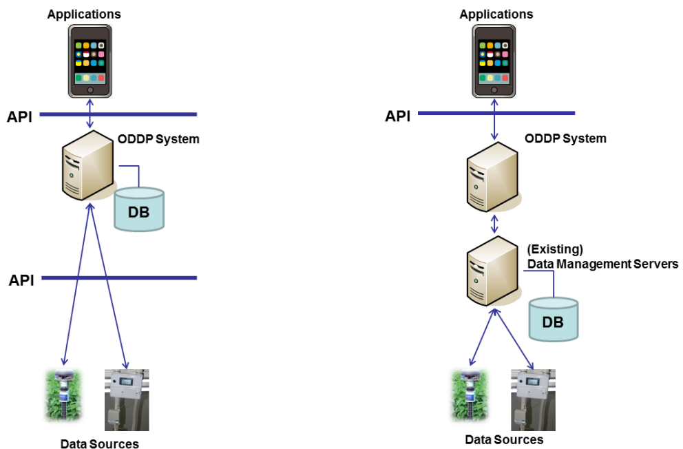
(a) 情報源・アプリケーションともに ODDP API に準拠 (b) 既存のデータ処理システムに ODDP API を付与
