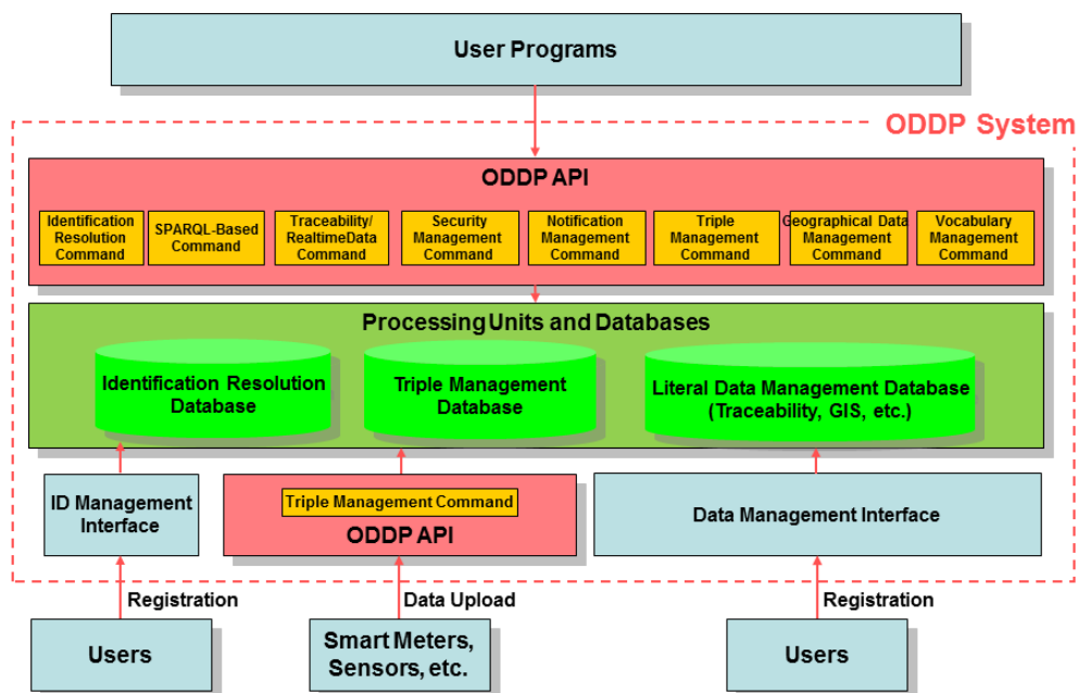
図 3.1: 情報流通連携基盤システムの構成
