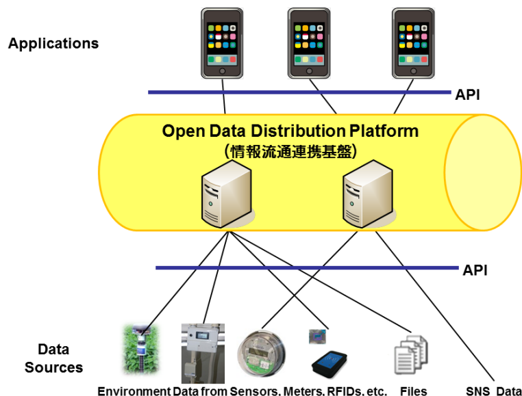
図 1.1: 情報流通連携基盤の全体像
